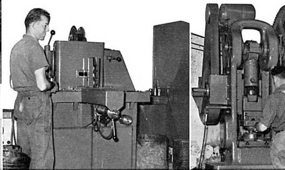
Ci-dessus : M. COLLAVERI, Préfet de la Loire, reçoit des mains de M. Georges SOUVIGNET un coffret de boules SUPERINOX OBUT. Voici par ailleurs, le four et les bacs de chromage. Ci-Cont.e : la machine automatique à souder les boules, une presse et les tours.
